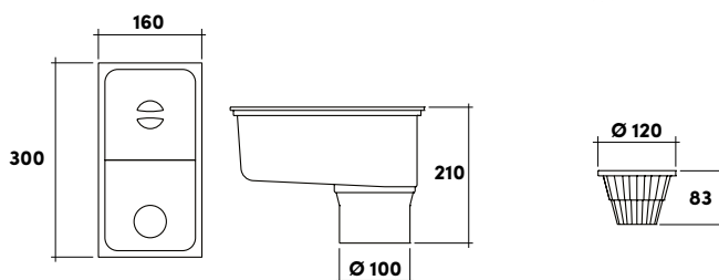
Pozzetto pluviale con uscita verticale Regenablauf mit vertikalem Ausgang
